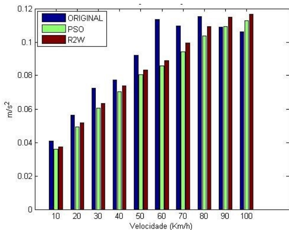
Fig. 2: RMS da aceleração vertical na cabeça do Motorista no Asfalto A. Fonte: Autor
